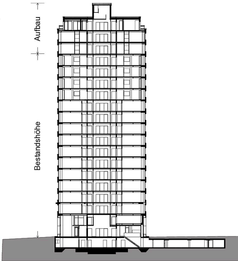
Systemschnitt II Neu
