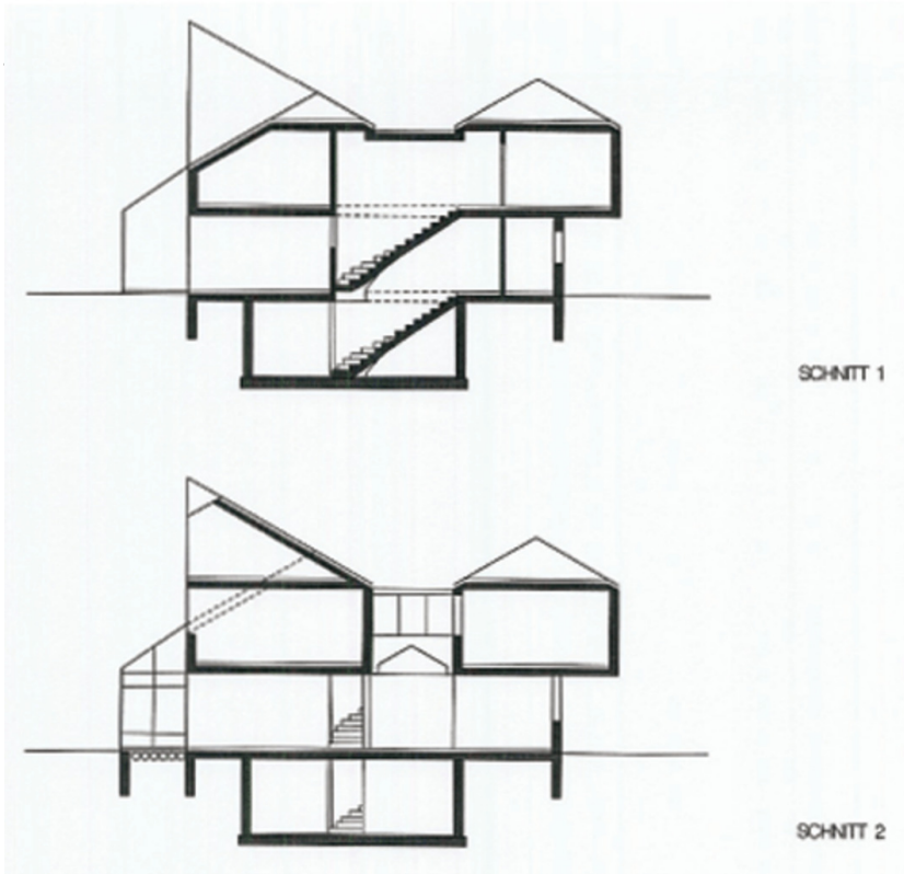
Schnitt
