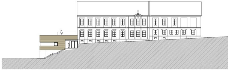
ANSICHT OSTEN
