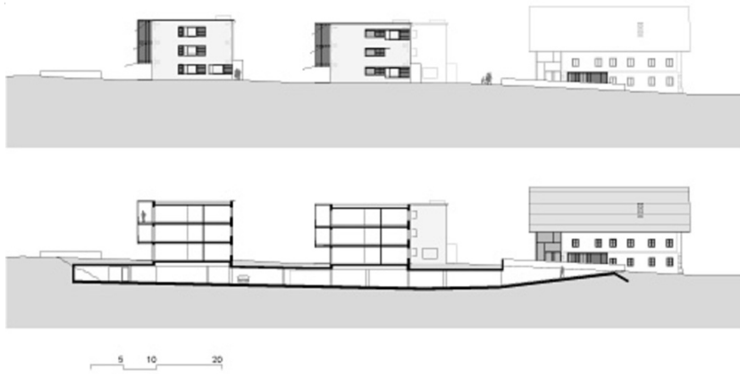
Ansicht schnitt
