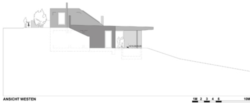
ANSICHT WESTEN
