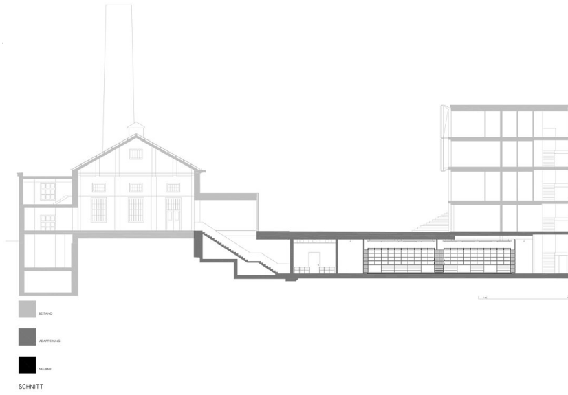
Kesselhaus, Schnitt
