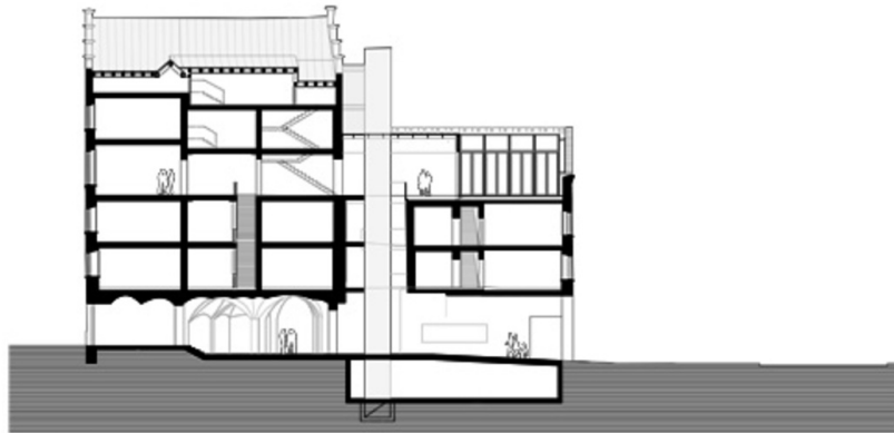
LANGSSCHNITT
