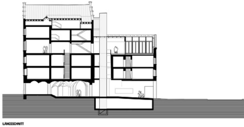
Längsschnitt
