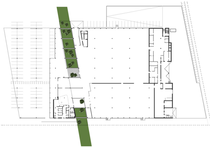
GRUNDRISS ERDGESCHOSS
