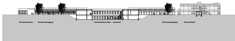
Schnitt bzw. Ansicht Süd
