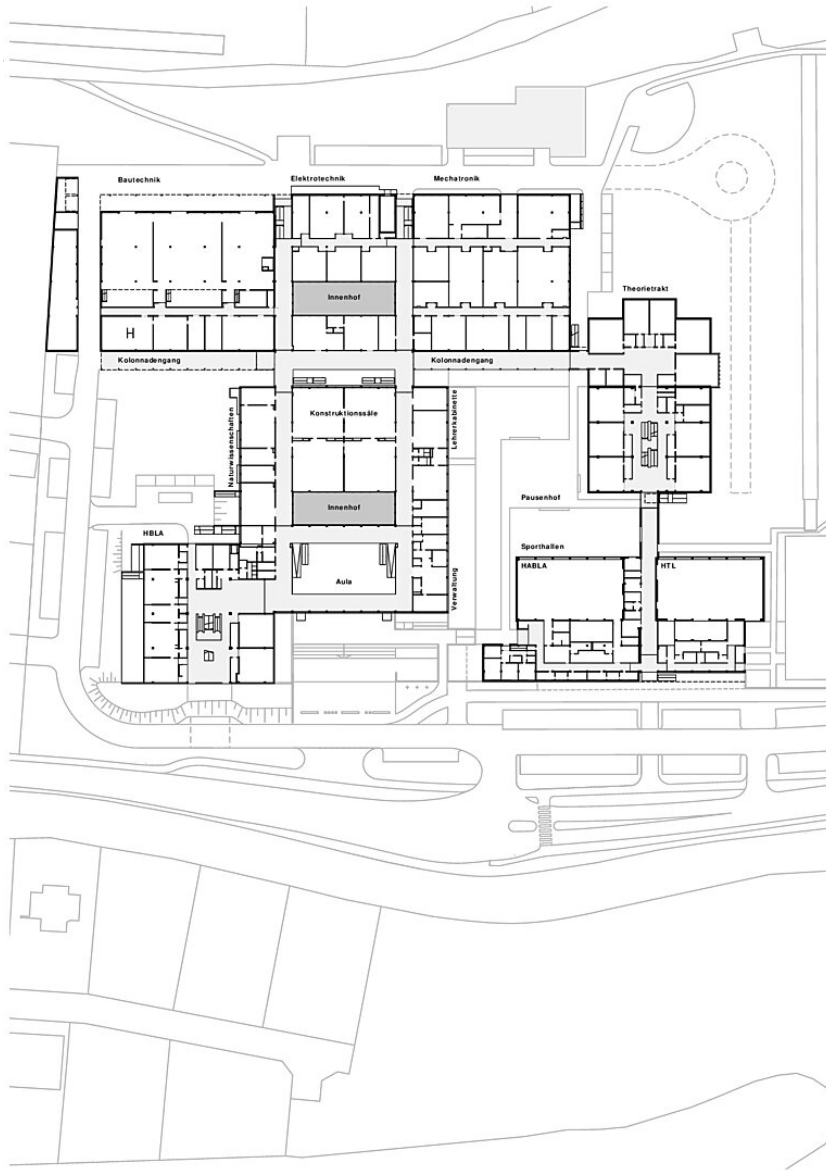
Grundriss Erdgeschoss
