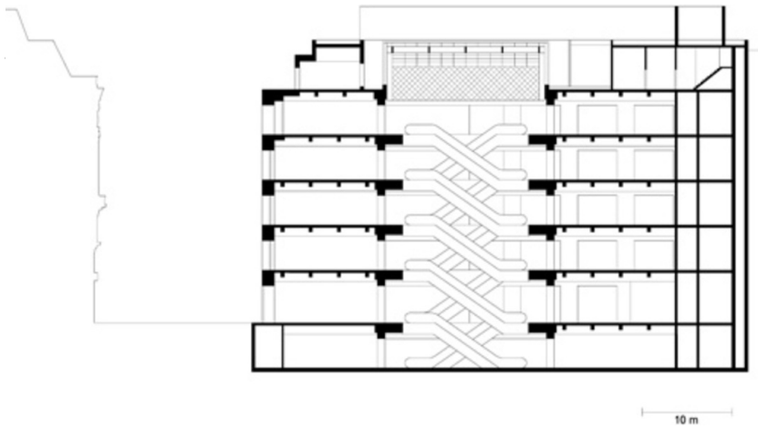
Längsschnitt
