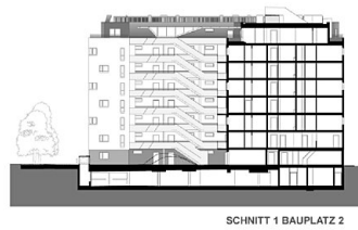
SCHNITT 1 BAUPLATZ 2
