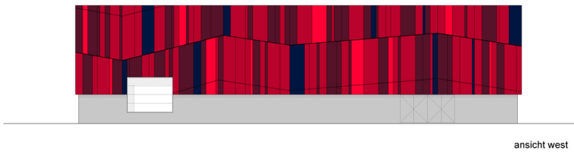
ansicht west
