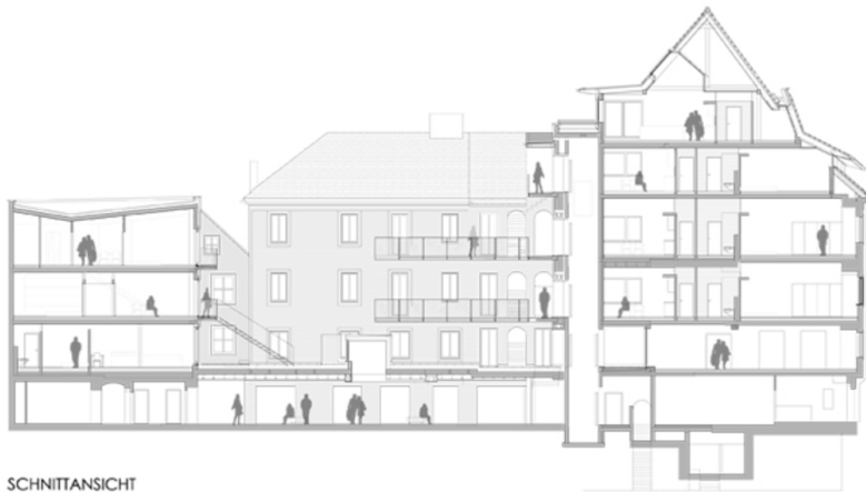
SCHNITTANSICHT
