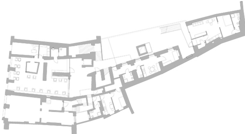
GRUNDRISS 1.OG
