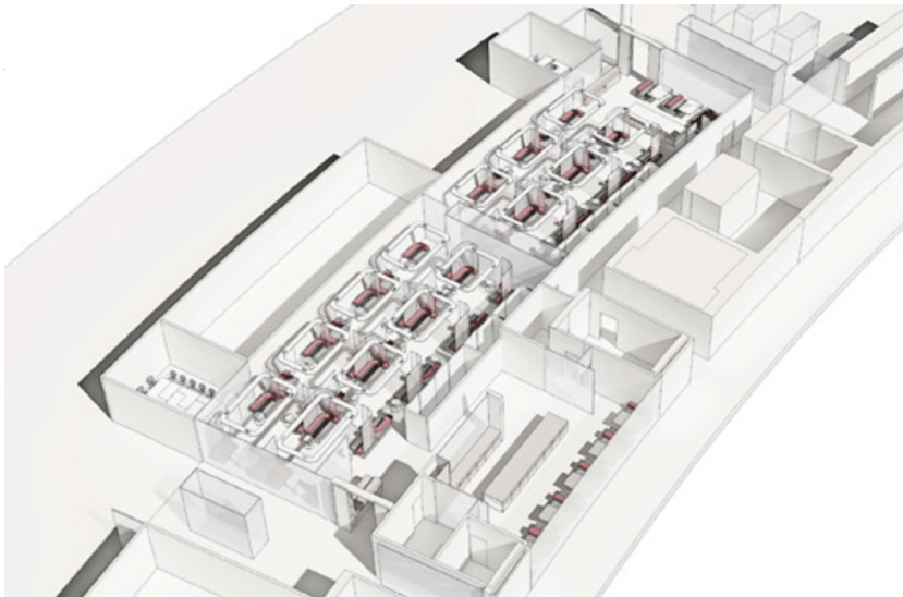
Axonometrie
