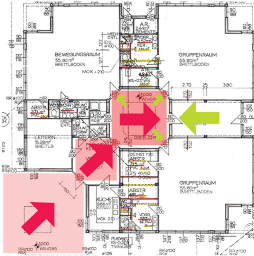
Grundriss Bestand
