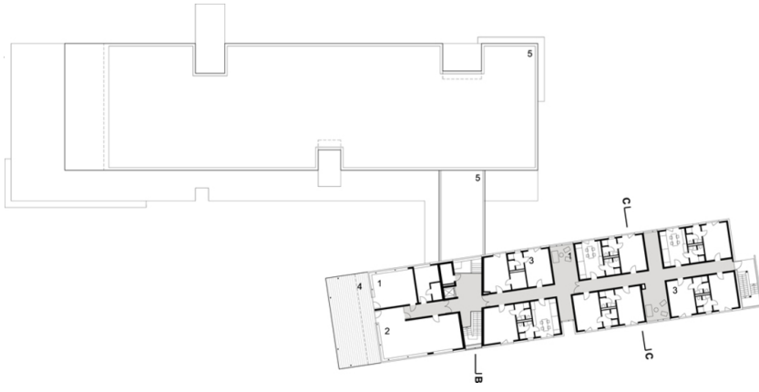
Grundriss OG2
