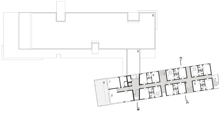
Grundriss OG2
