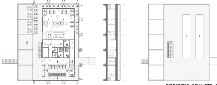
GRUNDRISS SCHNITTE 1:200
