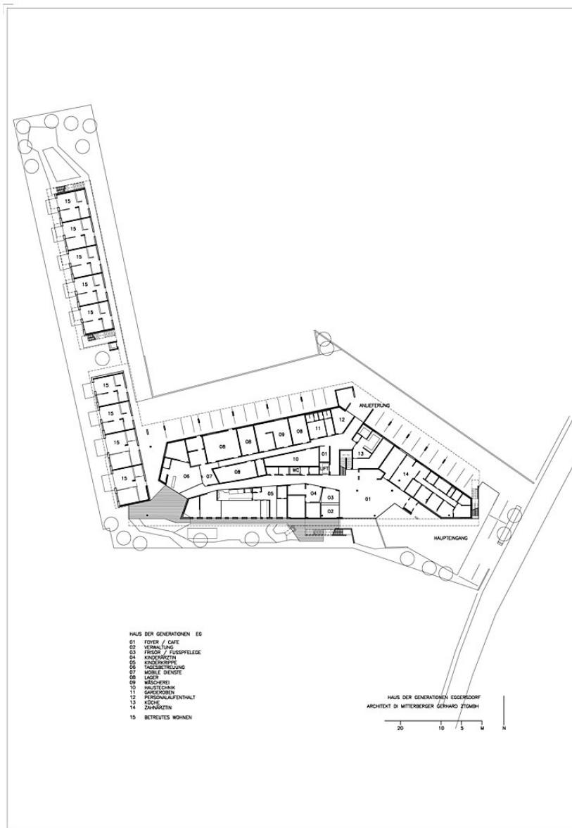
Grundriss Erdgeschoss
