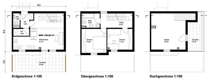
Erdgeschoss 1:100
