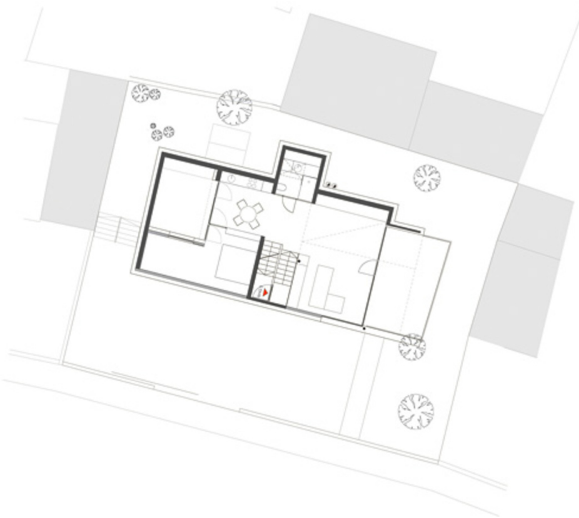
Grundriss DG
