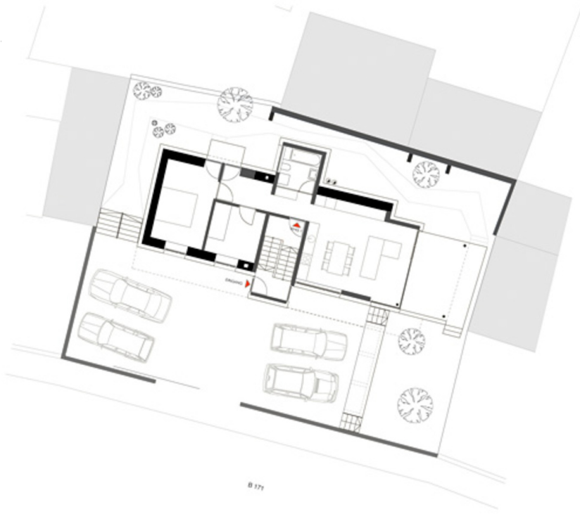
Grundriss EG
