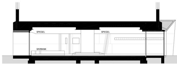
Schnitt B-B 1:100
