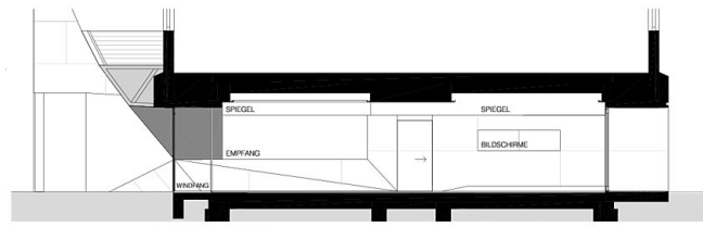
Schnitt A-A 1:100
