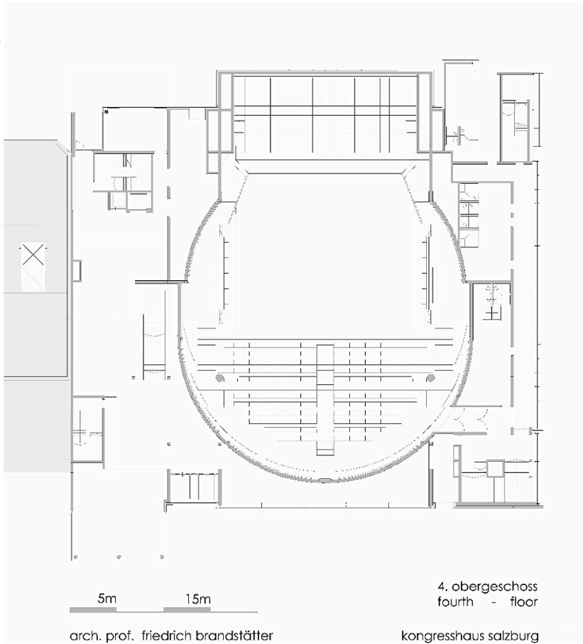
4. Obergeschoss
