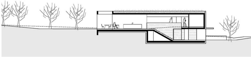
SCHNITT B
