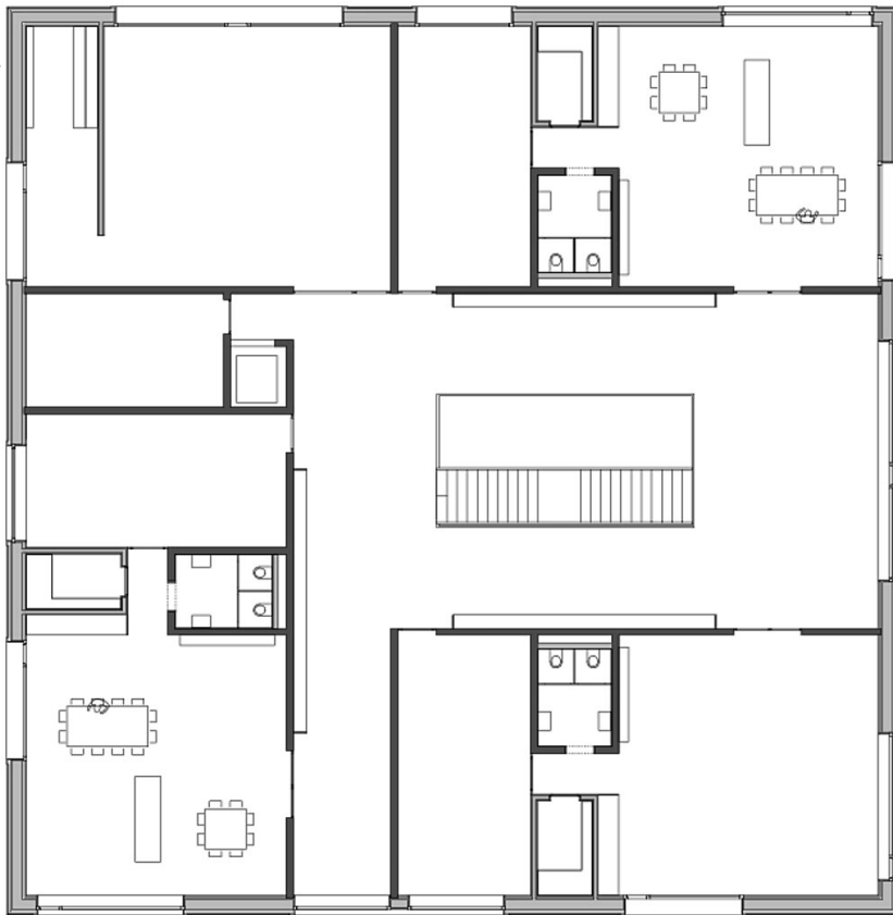
Grundriss Obergeschoss
