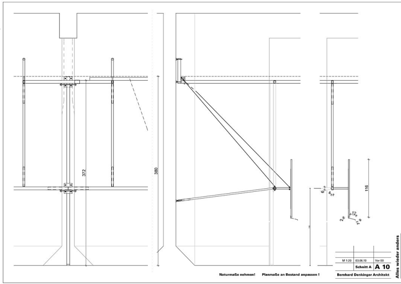
Tragkonstruktion zur Wand abgestützt
