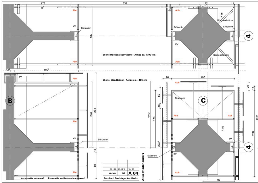
Horizontalschnitt Klemmverbindungen
