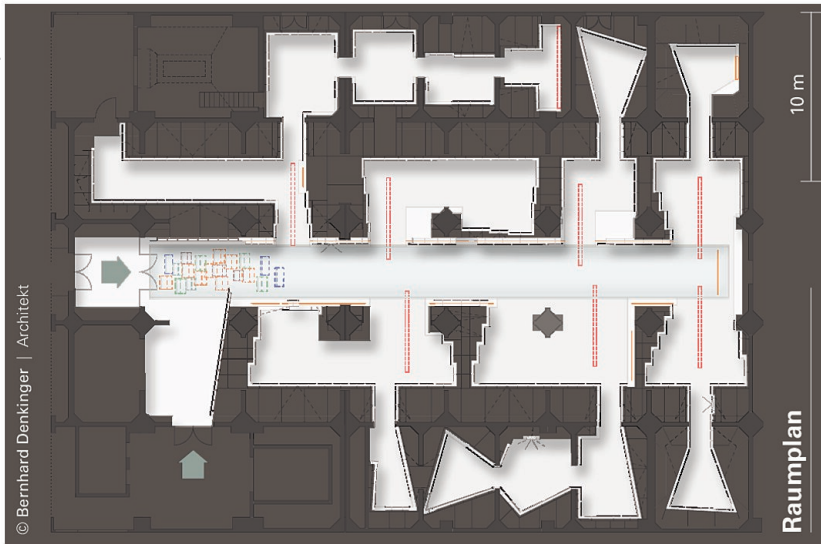
Grundriss
