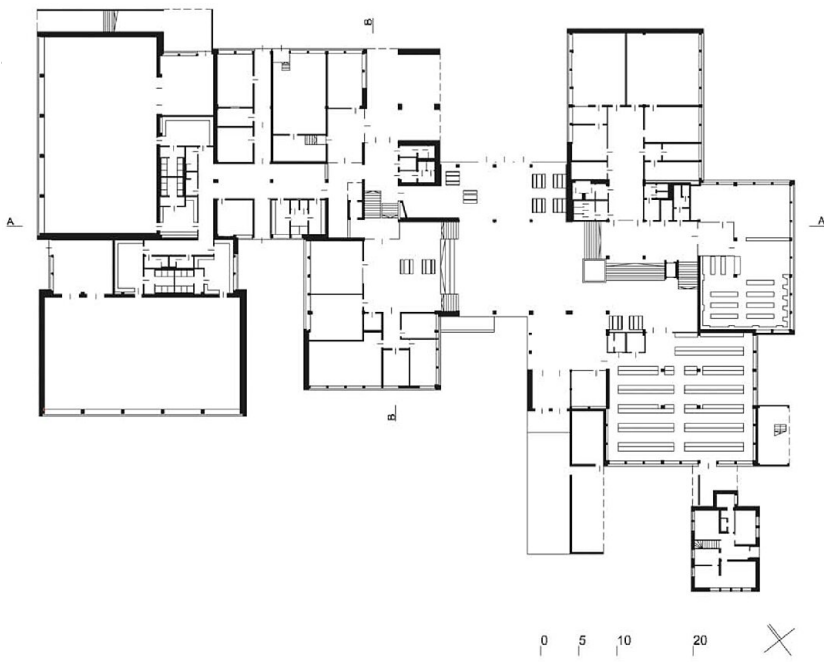
Grundriss Erdgeschoss
