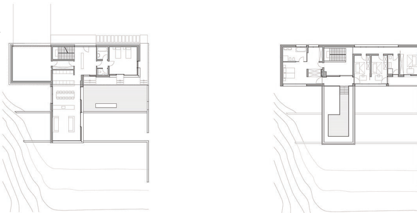
Erdgeschoß 1. Obergeschoß
