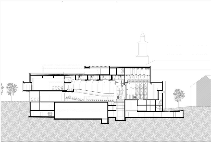
Schnitt A-A
