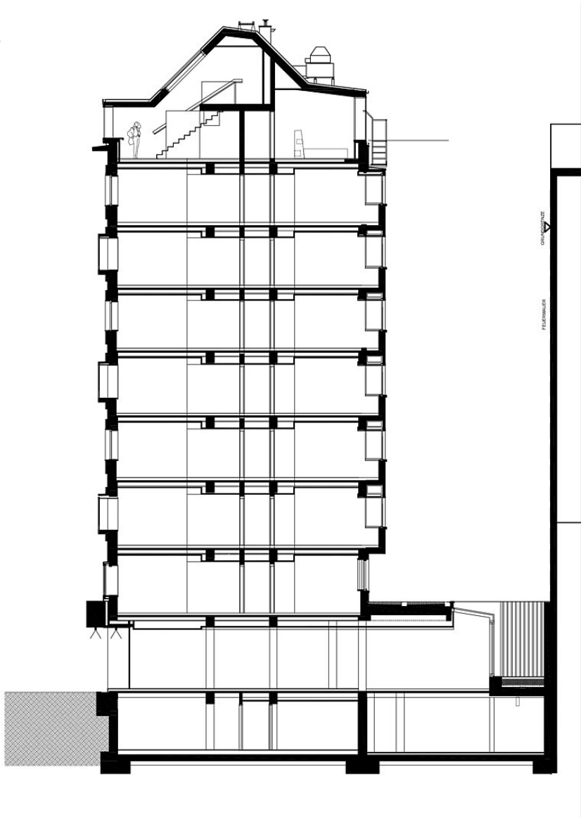
Schnitt
