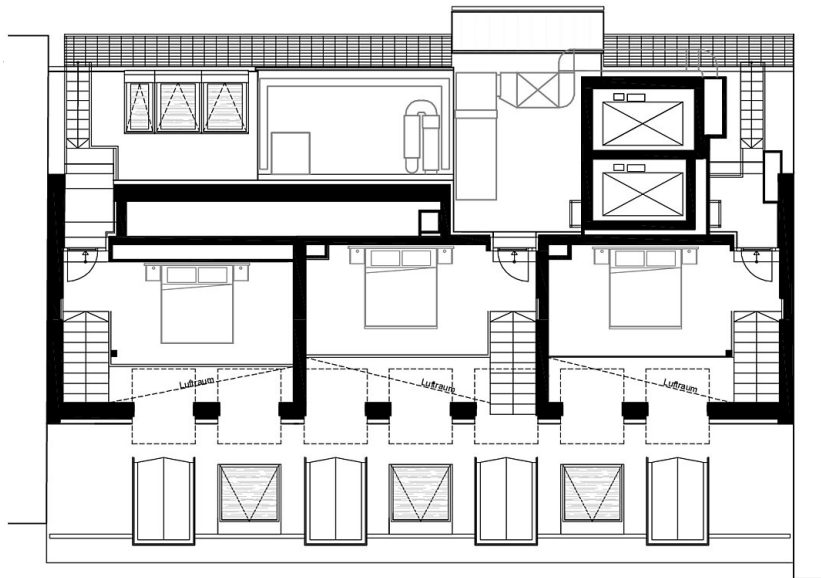
Grundriss Galeriesgeschoss
