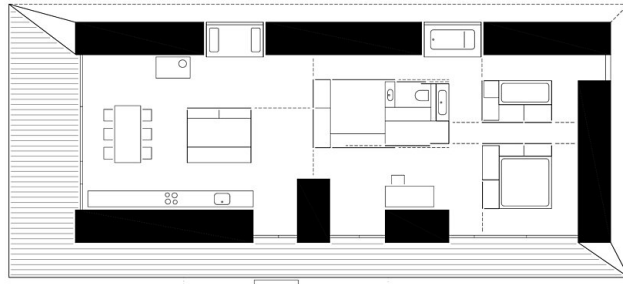
Lasttragendes Strohhaus
