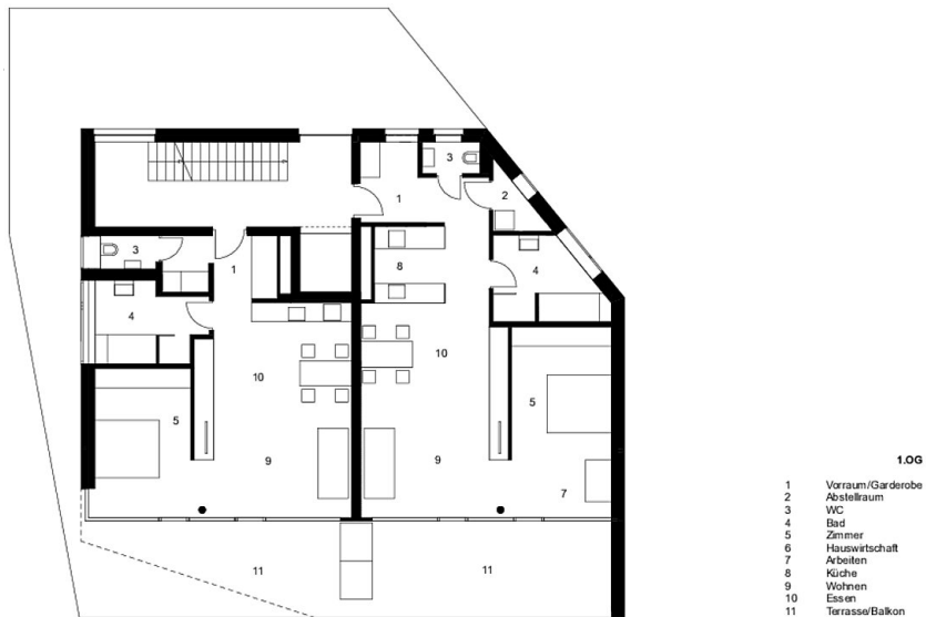
Grundriss OG1
