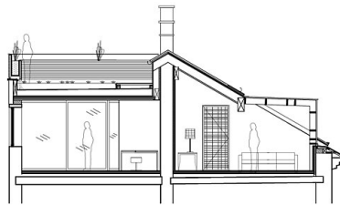
QUERSCHNITT, 1:100
