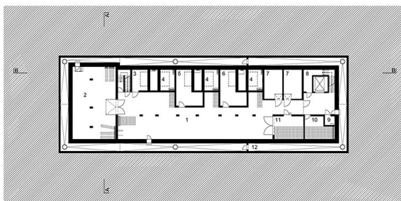
Grundriss 3, Untergeschoss (G01)
