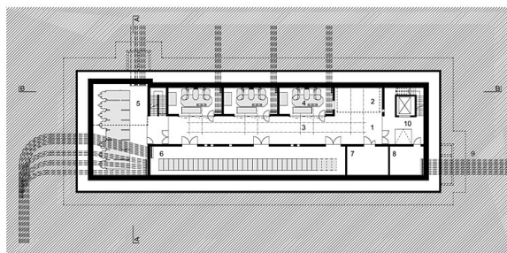
Grundris 2, Untergeschoss (G02)
