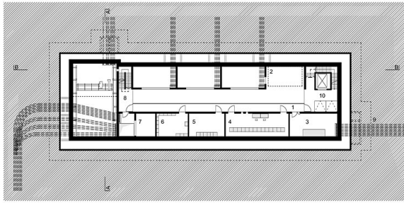
Grundriss 1, Untergeschoss (G00)
