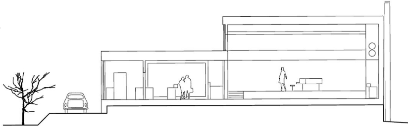
Schnitt A-A 10 11 12 15 19
