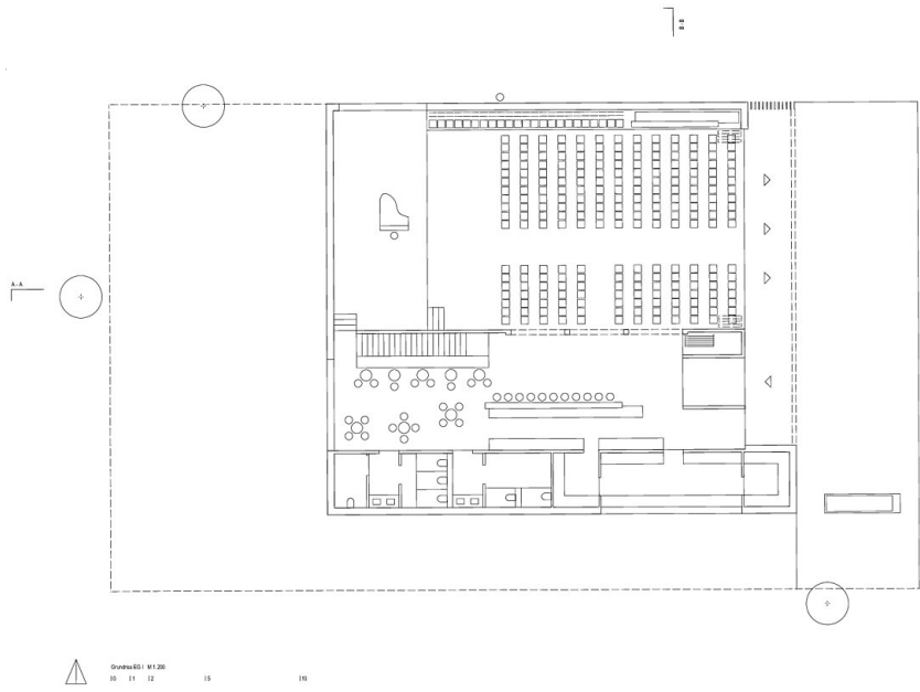
Grundriss EG
