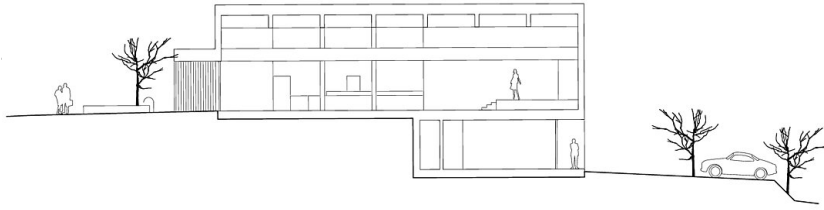
Schnitt A-A 10 11 12 15 19
