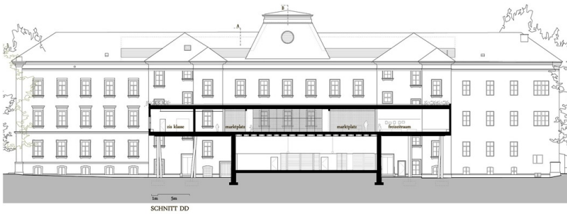
1cm 5m SCHNITT DD
