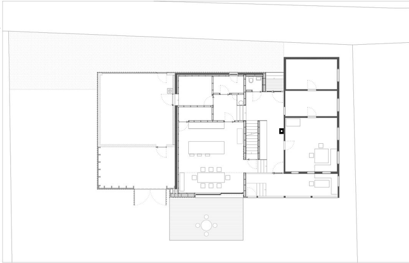
Erdgeschoß
