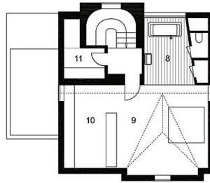
Grundriss Dachgeschoss
