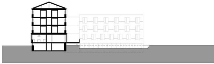
SCHNITT D-D
