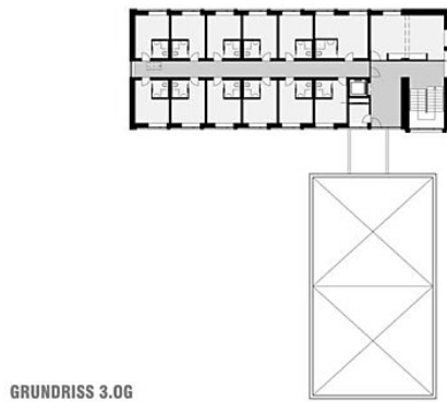
GRUNDRISS 3.OG
