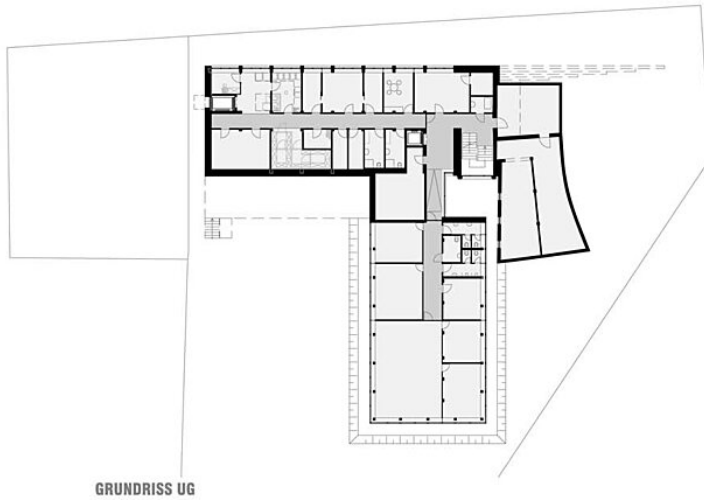
GRUNDRISS UG
