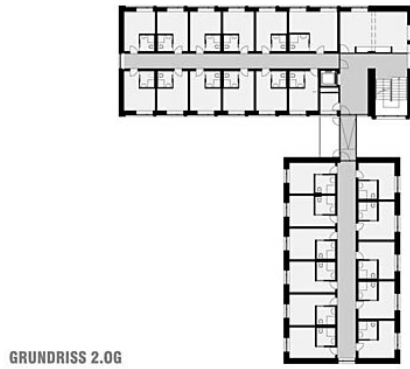
GRUNDRISS 2.OG
