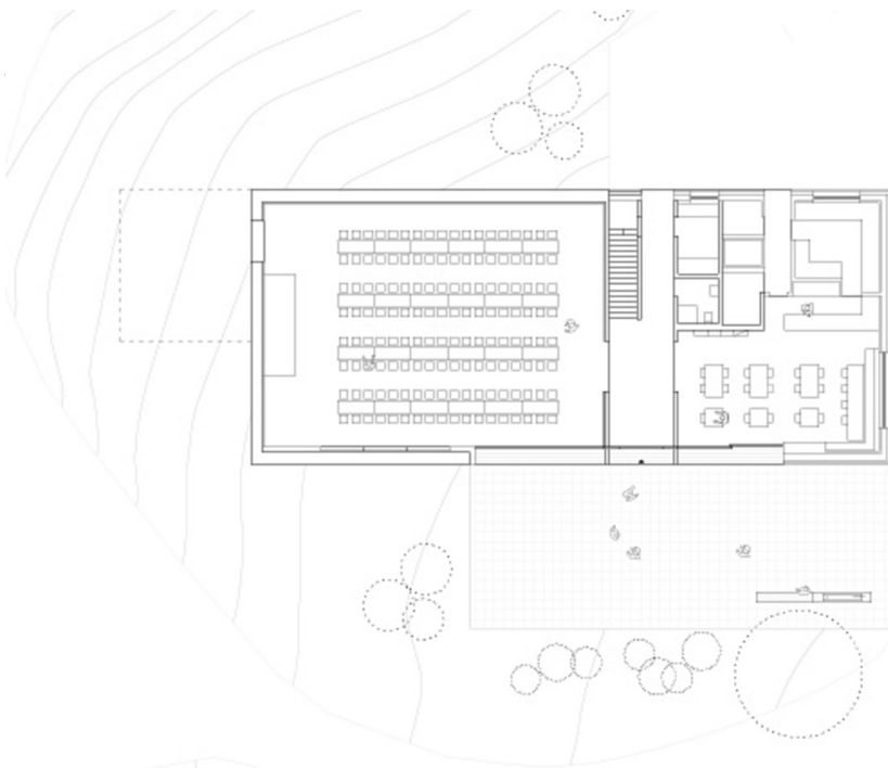
Grundriss
