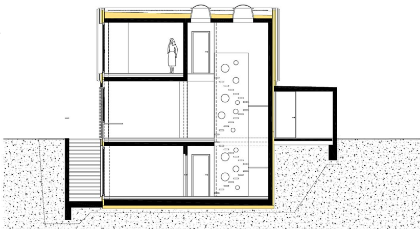
Schnitt AA
