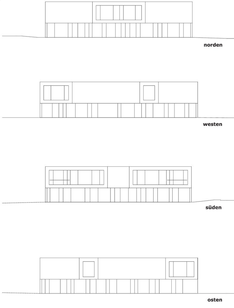
Ansichten
