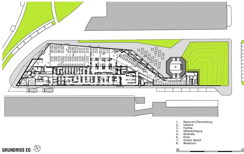
Grundriss EG
