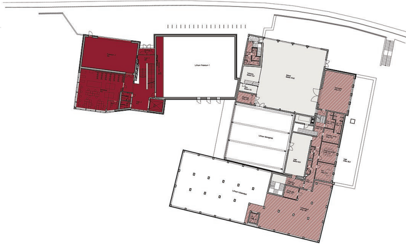
Grundriss OG1
