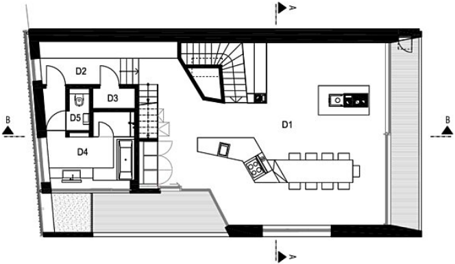
Grundriss Dachgeschoss
