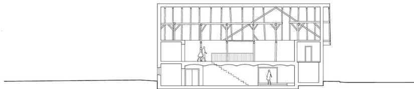
Schnitt B-B | M 1:200 | 0 | 1 | 1 | 2 | 5 | 10
