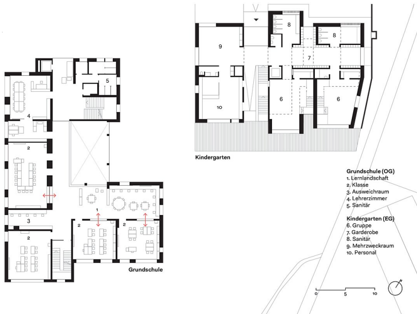
Grundriss OG-EG
