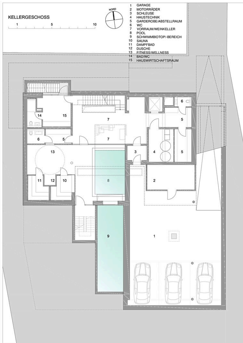
Grundriss Keller
