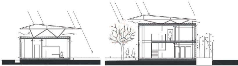
Querschnitt Konzeptdarstellung
