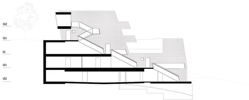
SCHNITT A-A 1:200
