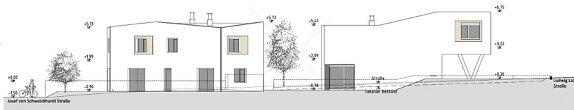
Ansicht SO
